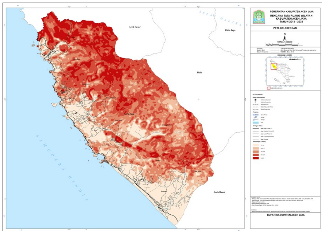
Gambar 2.2 Peta Kemiringan Lahan Kabupaten Aceh Jaya
